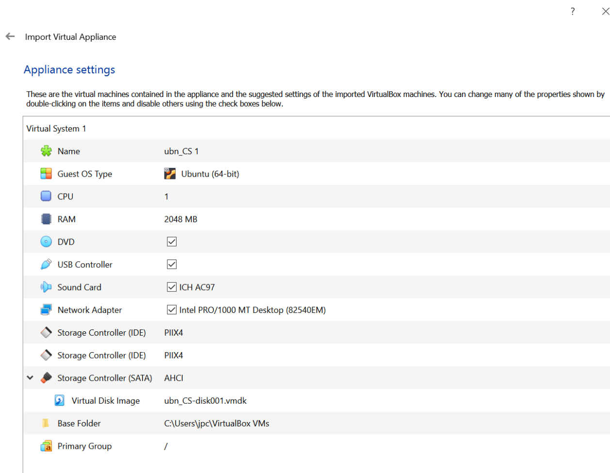
Рисунок 3 Свойства виртуальной машины
